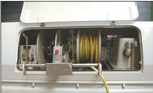
Hydraulische HDschlauchtrommel Aufnahme von 80 m 3/8" Schlauch Füllschlauchtrommel
