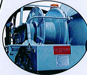
150 m 1" (oder 100m 3/4") schwenkbare Tommel mit manueller Schlauchführung
