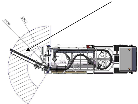
Evolu Eco Pack 2 + (avec bras télescopique)
