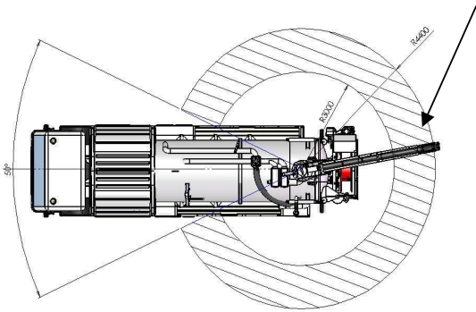
Combi pack + (avec flèche télescopique)
