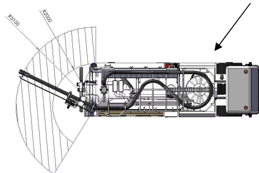
Evolu Eco Pack 2 + (avec bras télescopique)
