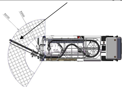
Evolu Eco Pack 2 + (avec bras télescopique)
