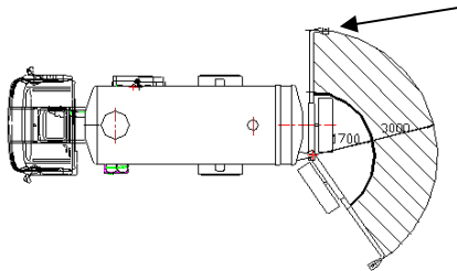
Combi pack + (avec orientation et translation)
